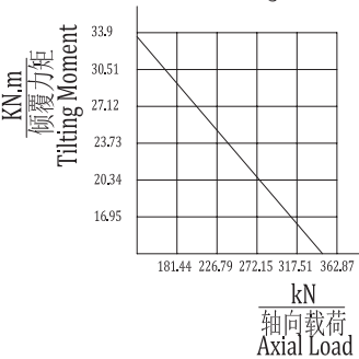
承载力矩图 MOMENT LOAD CHART
